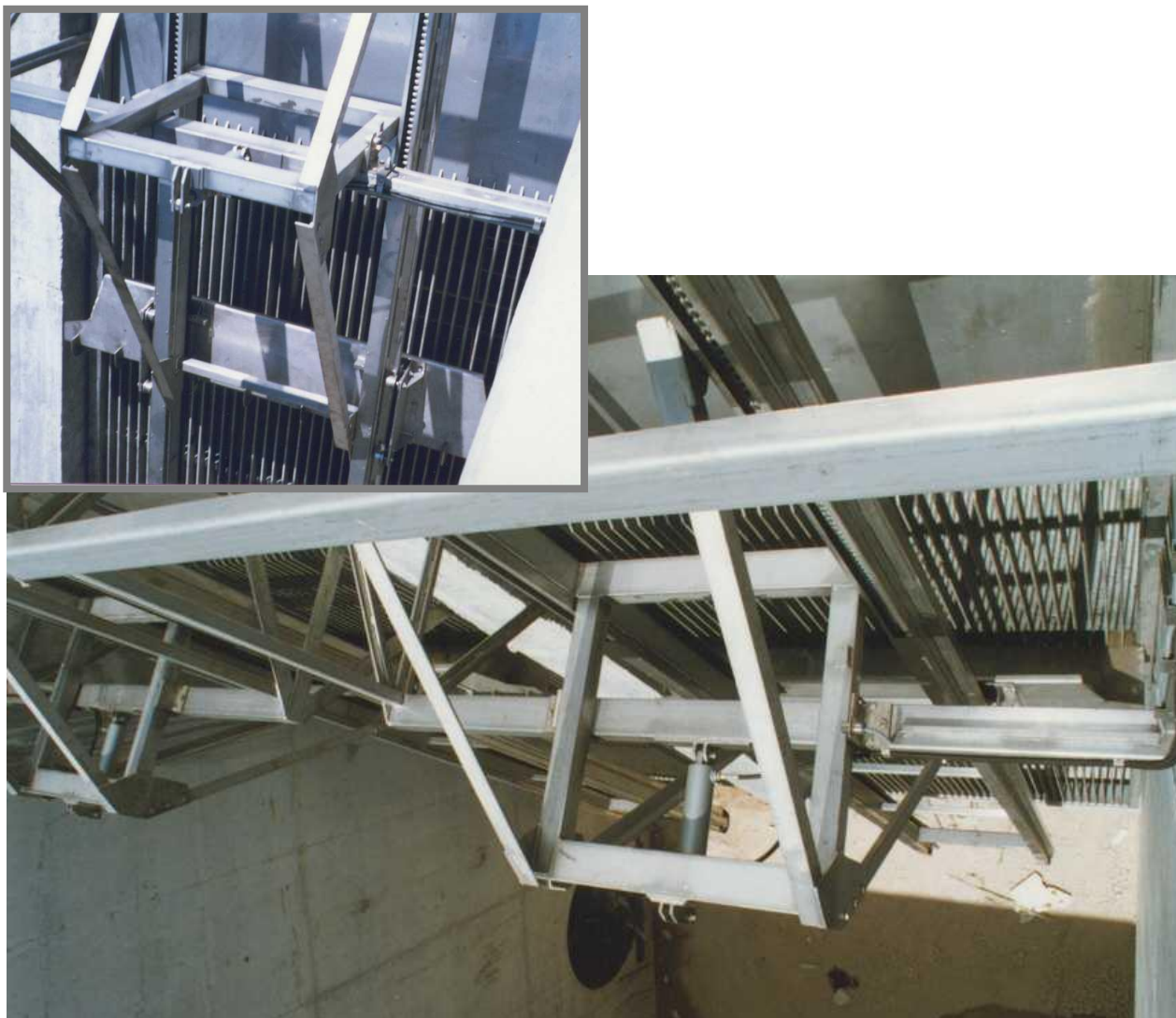
El balanceo de la estructura guía + carro porta-peine, lo efectúa un pistón hidráulico.
